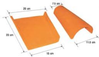
KL-011 กระเบื้องหลังคา ดินเผาลอนกลายกล้วยรุ่นแยกชิ้น
