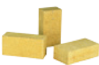
AR-132 อิฐทนไฟ SK-30 ขนาด 10x22.5x7.5 cm. 52 pcs./sqm. 3.2 kg.
